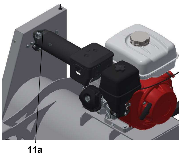
Obr. 11: Mazací body
