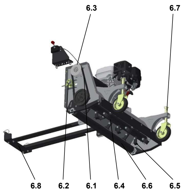
Obr. 6: Popis stroje pohled B
