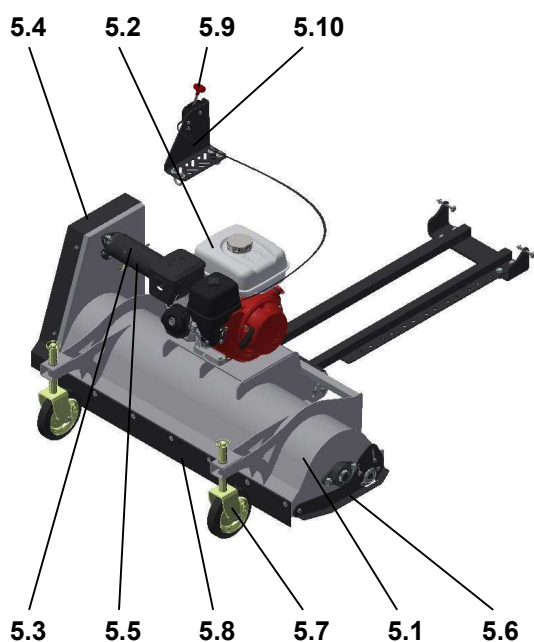
Obr. 5: Popis stroje pohled A
