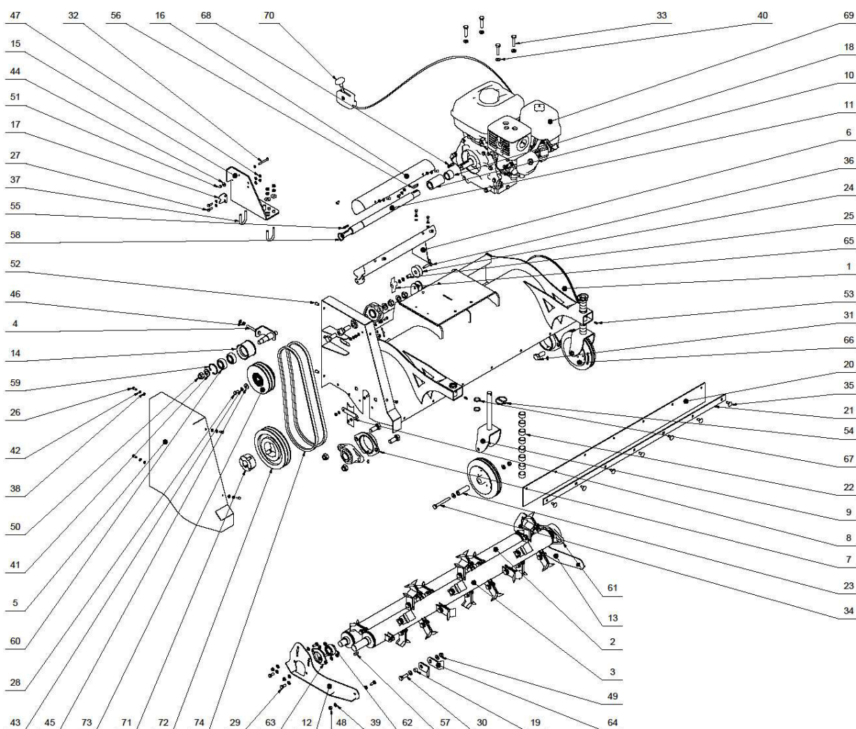
Obr. 14: Rozpad
